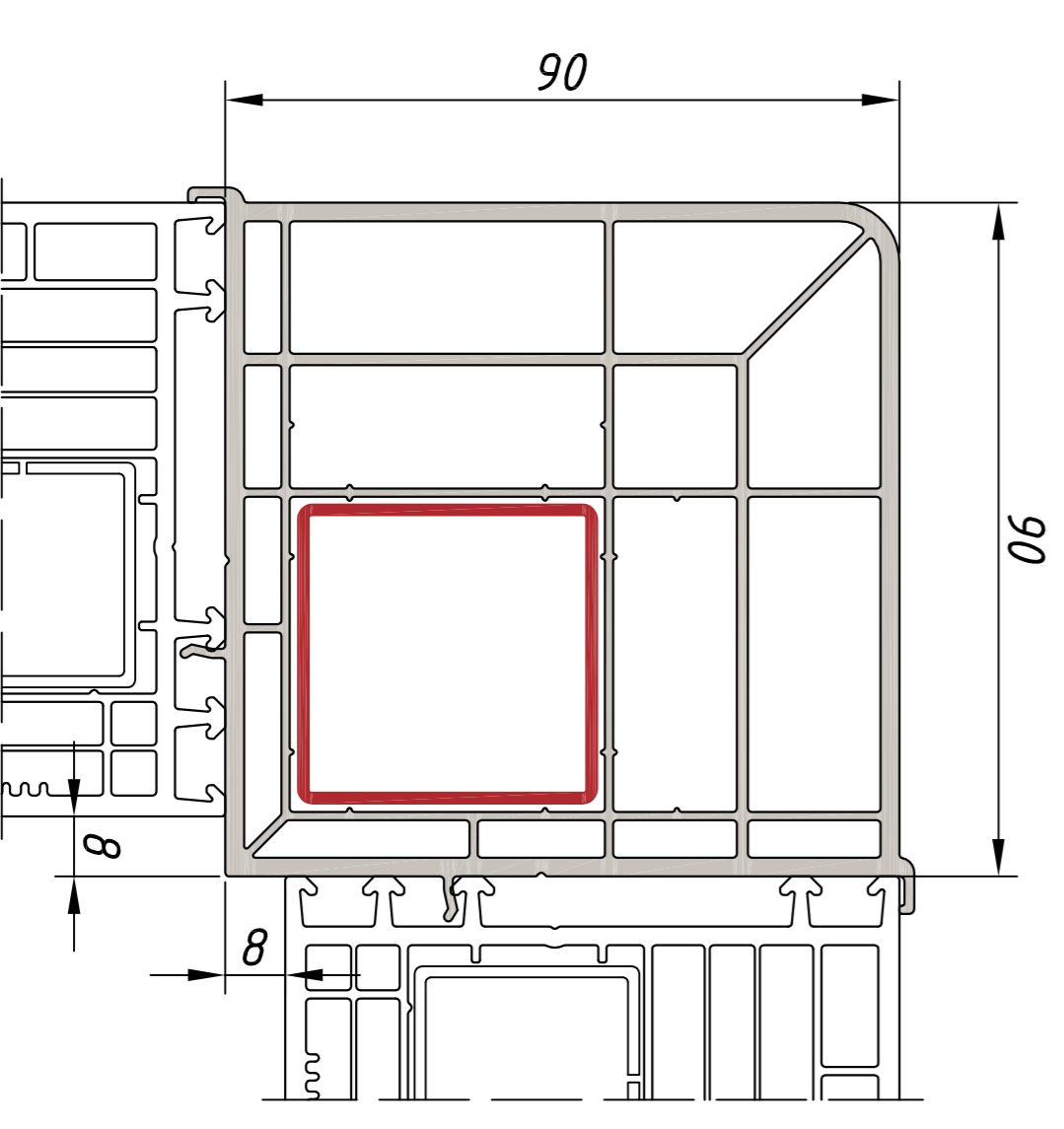
угловой соединитель 90гр арт. №116.214 усилитель арт. №13.281.2
