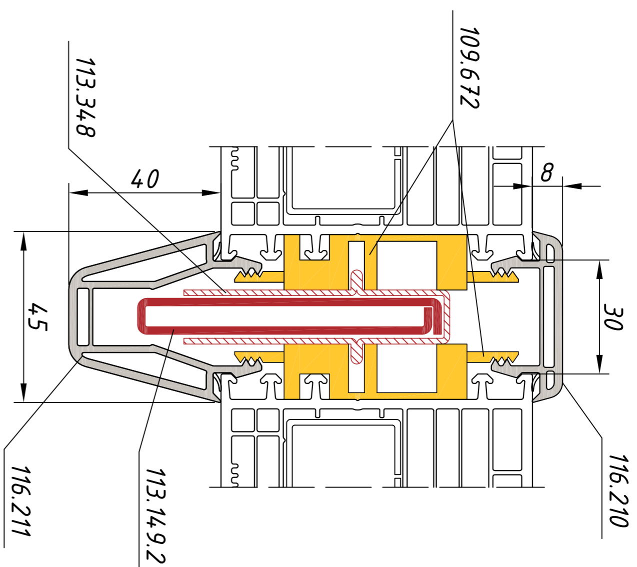
соединитель фасадный вертикальный соединитель 8x45 арт. №116.210 соединитель 40x45 арт. №116.211 усилитель арт. №13.348 усилитель арт. №13.1492 дистанционная вставка арт. №109.672 (шаг 4,00мм)
