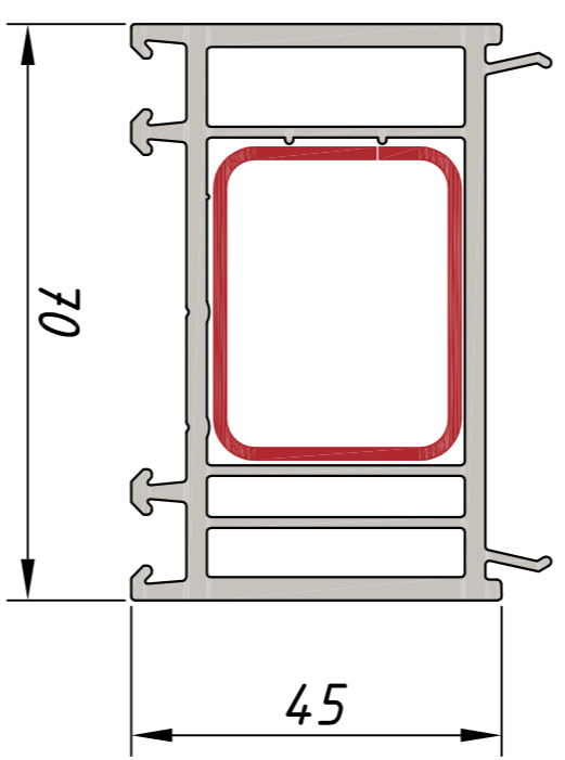
расширитель 45мм арт. №114.202 усилитель арт. №13.271
