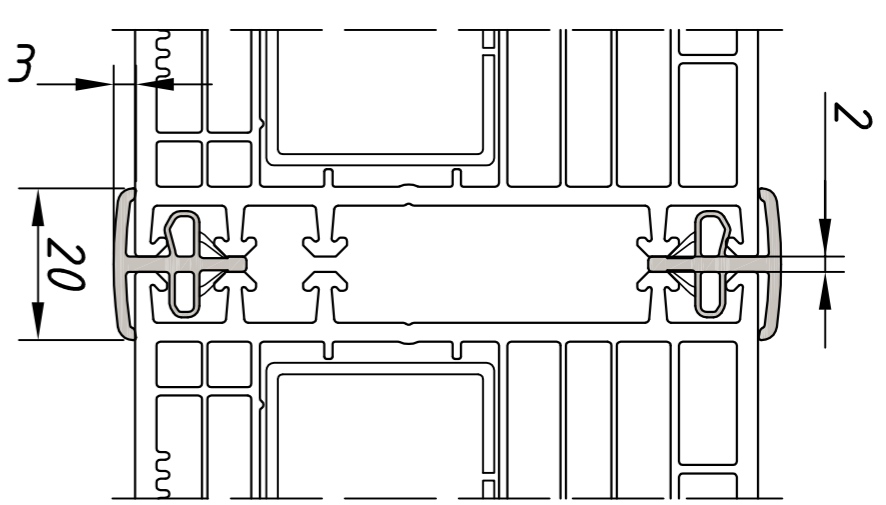
соединитель с уплотнением арт. №116.217 (2шт)
