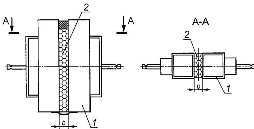
b - толщина шва; 1 - обойма из алюминия или нержавеющей стали толщиной 3 мм; 2 - образец испытуемого монтажного шва
