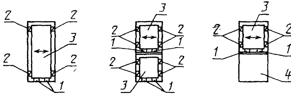
Двери со складывающимися полотнами
