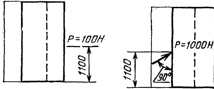
Дверь со складывающимися полотнами
