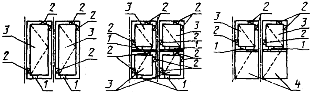
Двери со складывающимися полотнами
